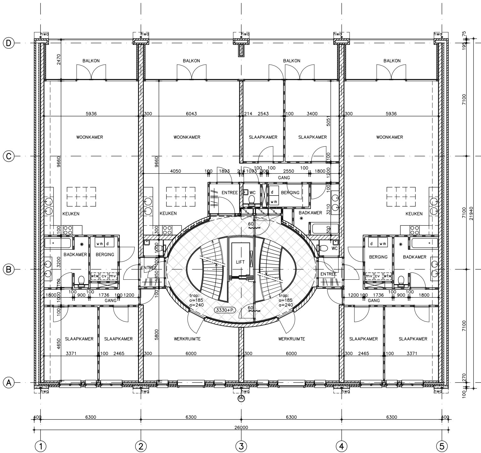
EERSTE VERDIEPING
