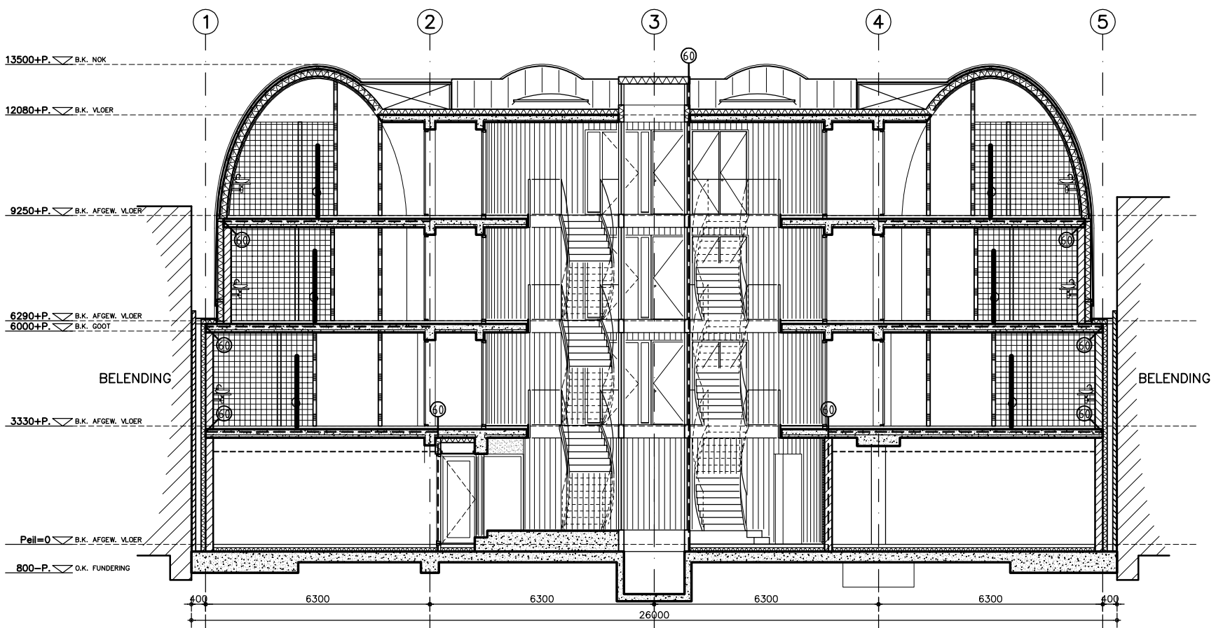
DOORSNEDE
