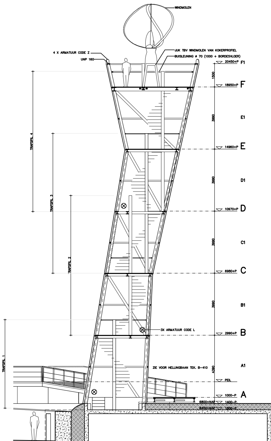
DOORSNEDE
