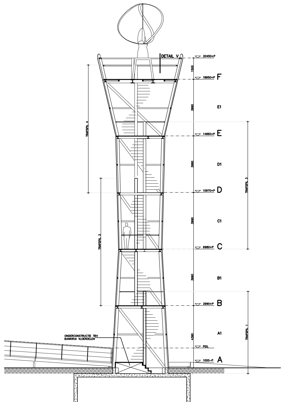
DOORSNEDE
