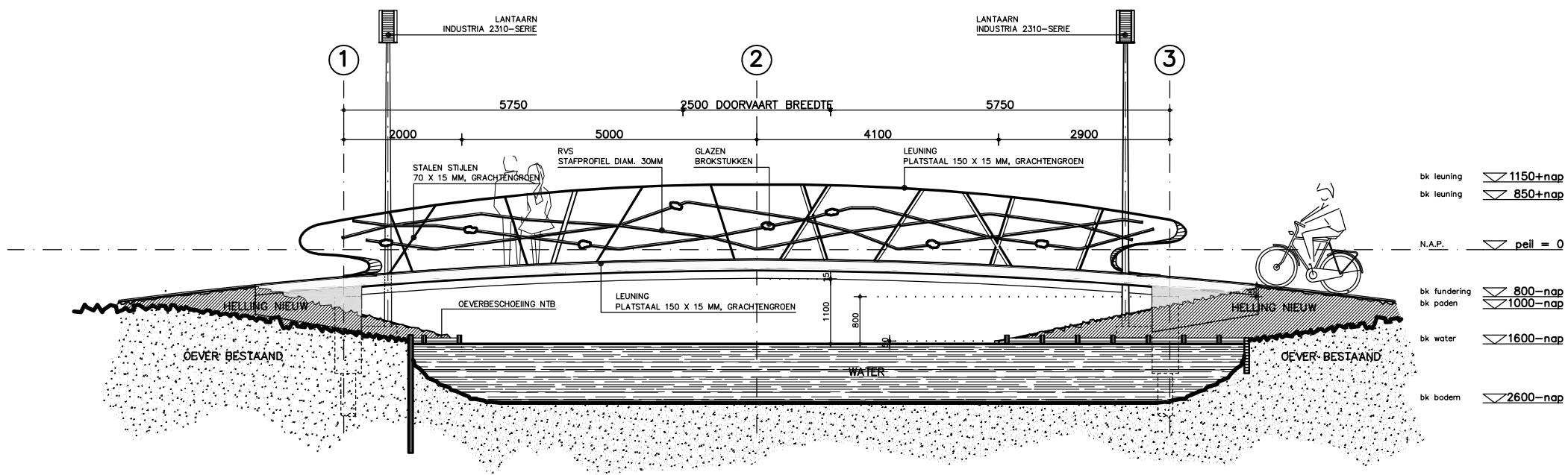
ZIJ-AANZICHT
