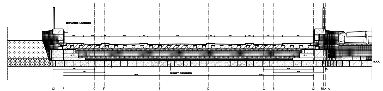
DOORSNEDE AA
