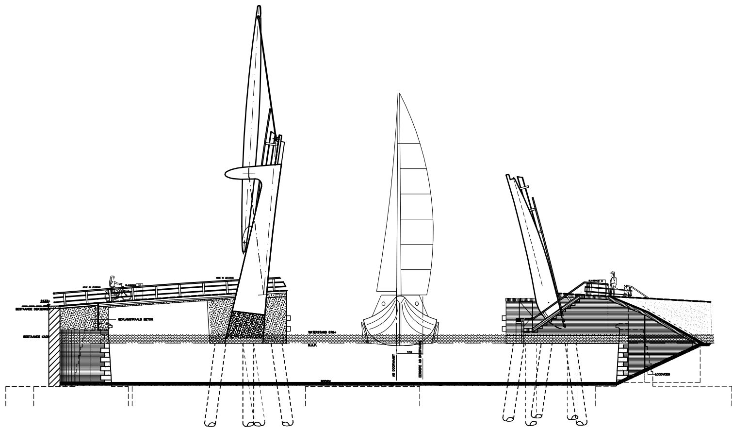
ZIJ-AANZICHT BRUGGEN
