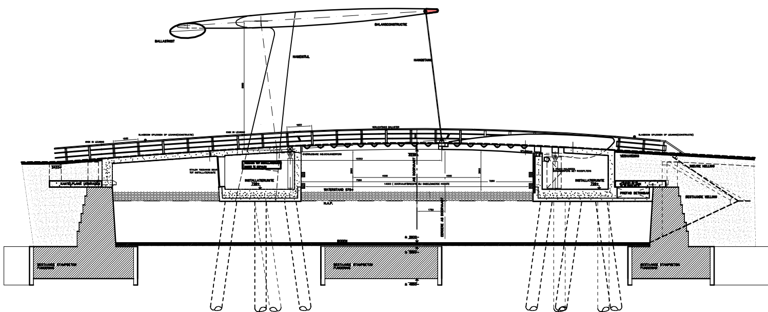
DOORSNEDE BRUGGEN
