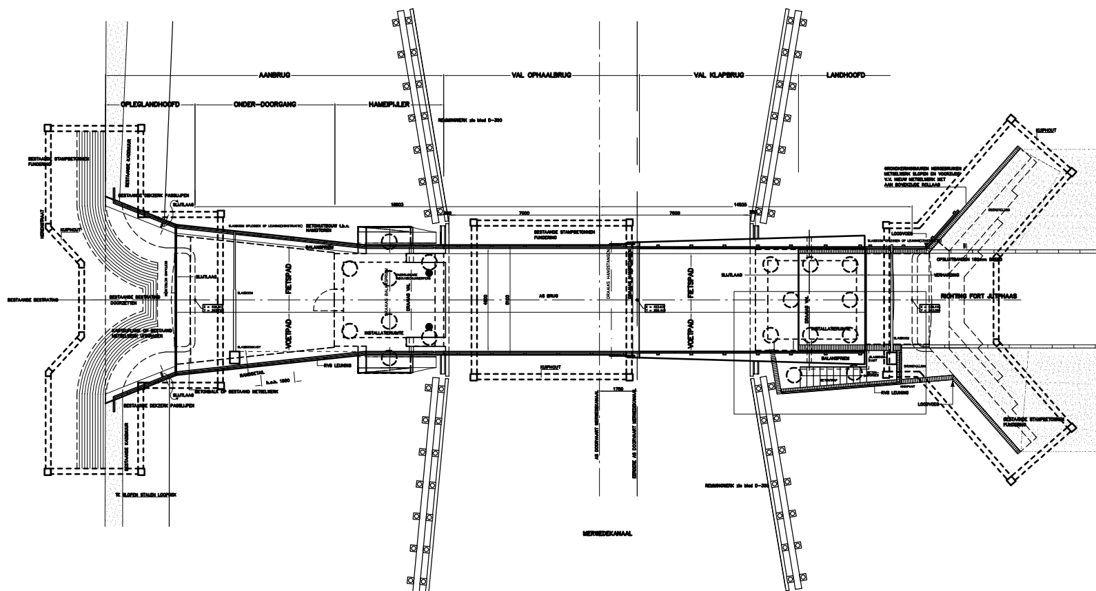
BOVENAANZICHT AANBRUG EN VALLEN
