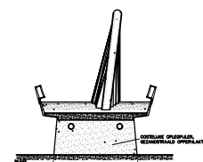
DOORSNEDE C
