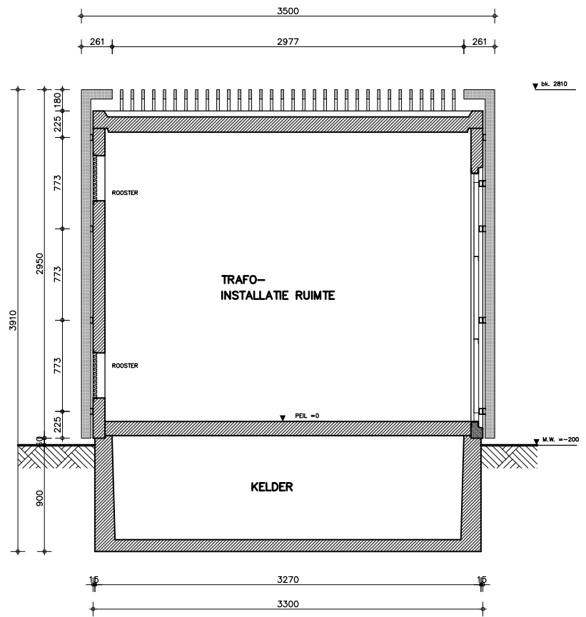
DOORSNEDE AA
