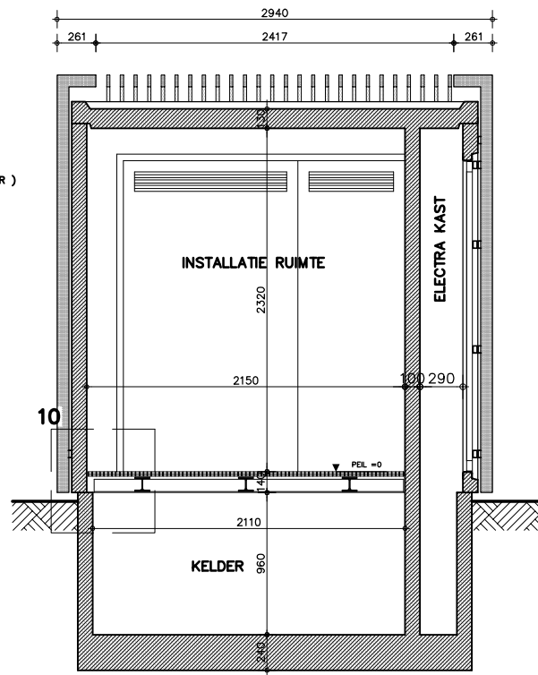
DOORSNEDE AA
