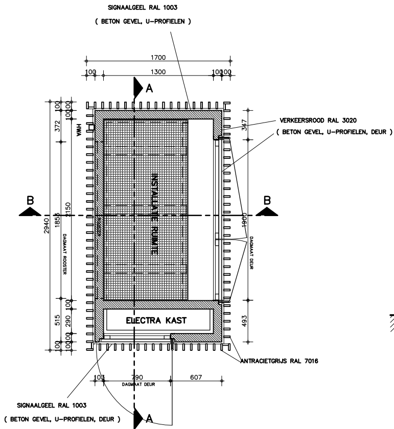
PLATTEGROND GASEXPANSIE
