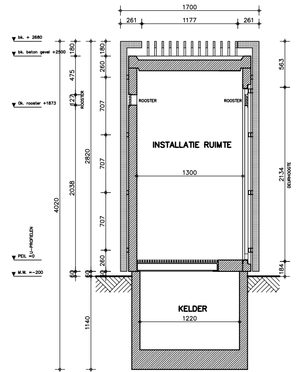
DOORSNEDE BB
