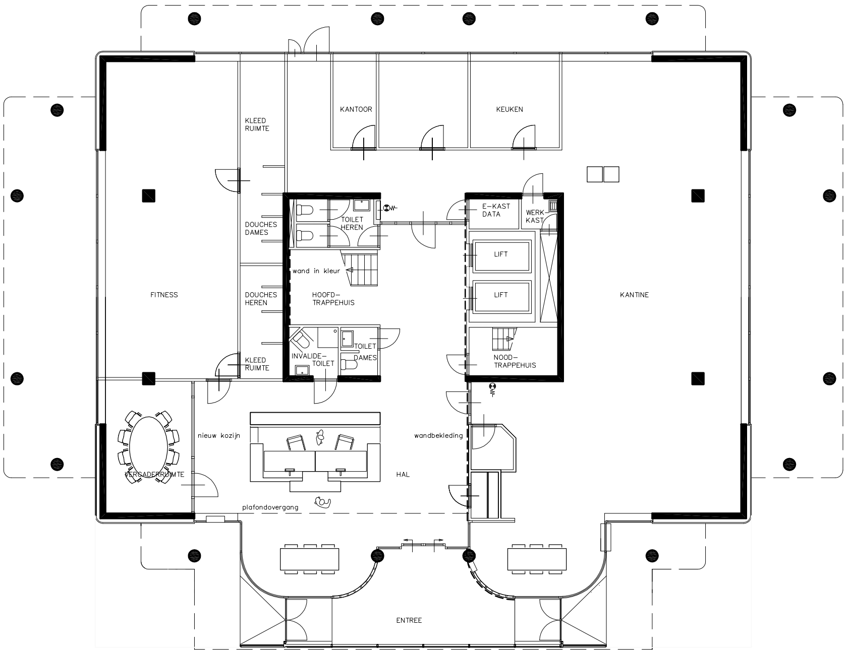
BEGANE GROND
