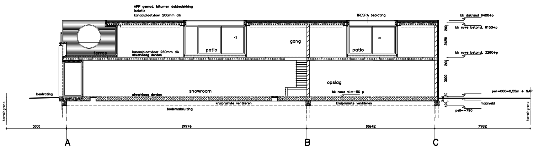
DOORSNEDE
