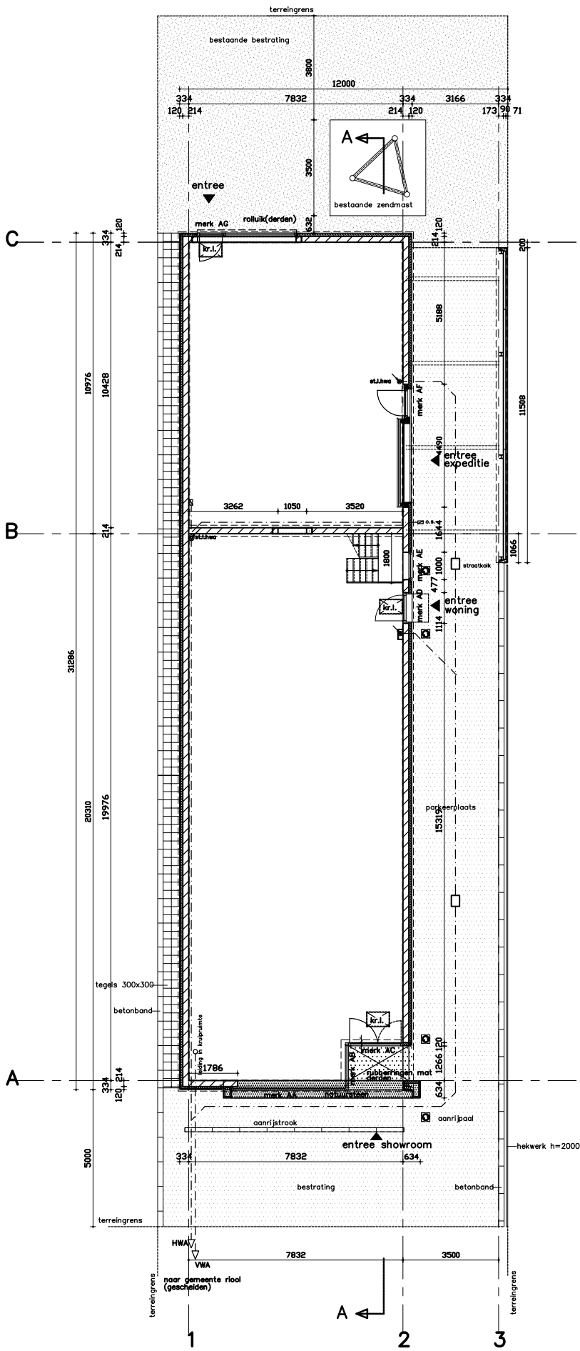
BEGANE GROND
