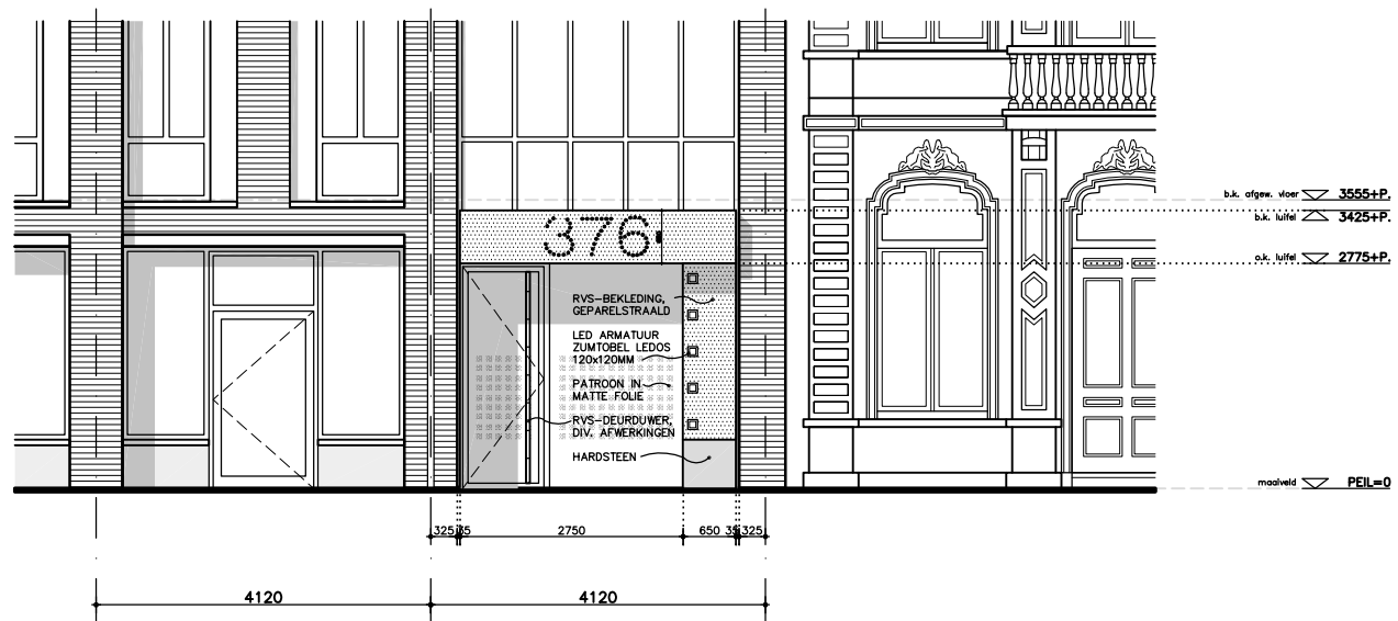
VOORGEVEL
