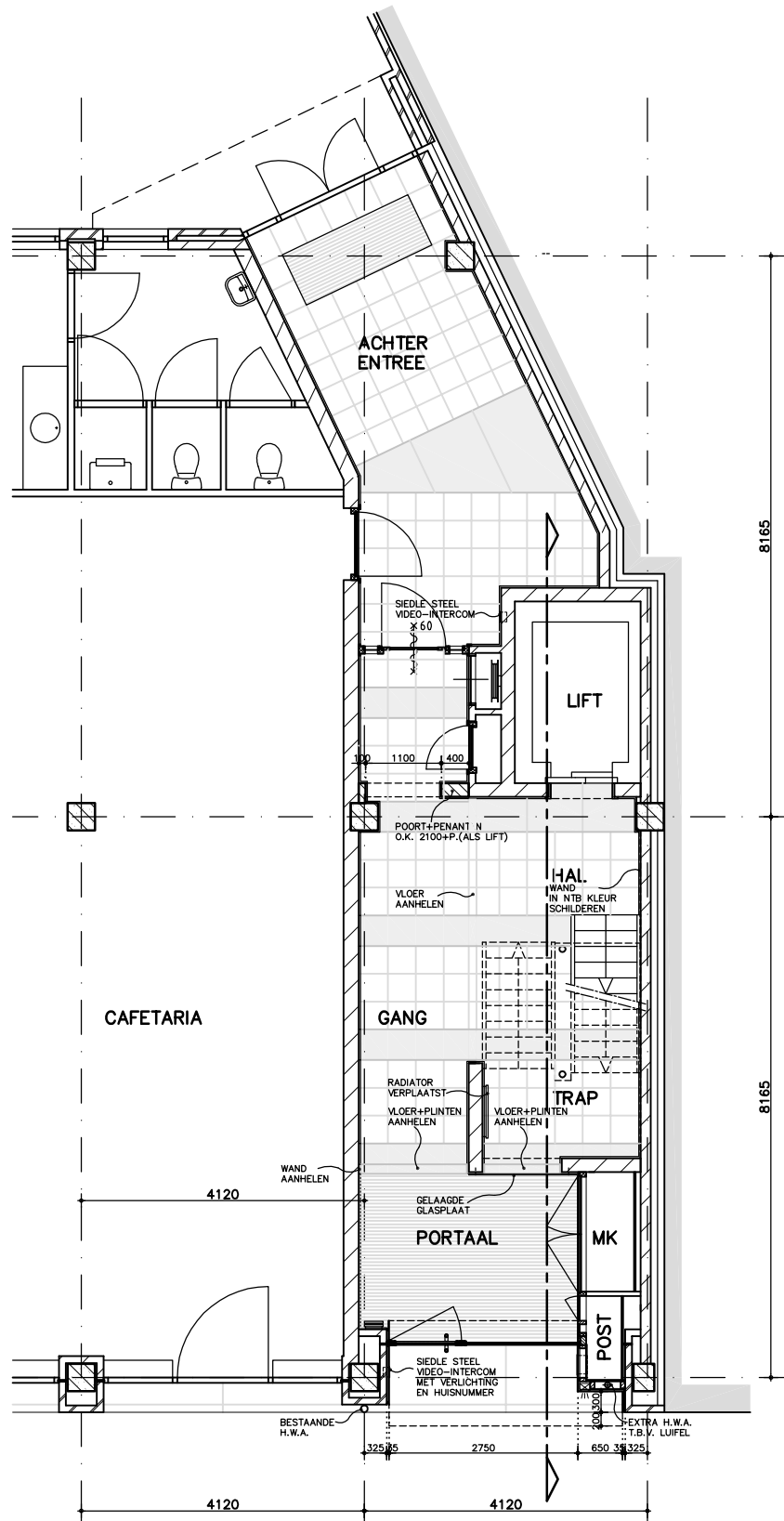
BEGANE GROND
