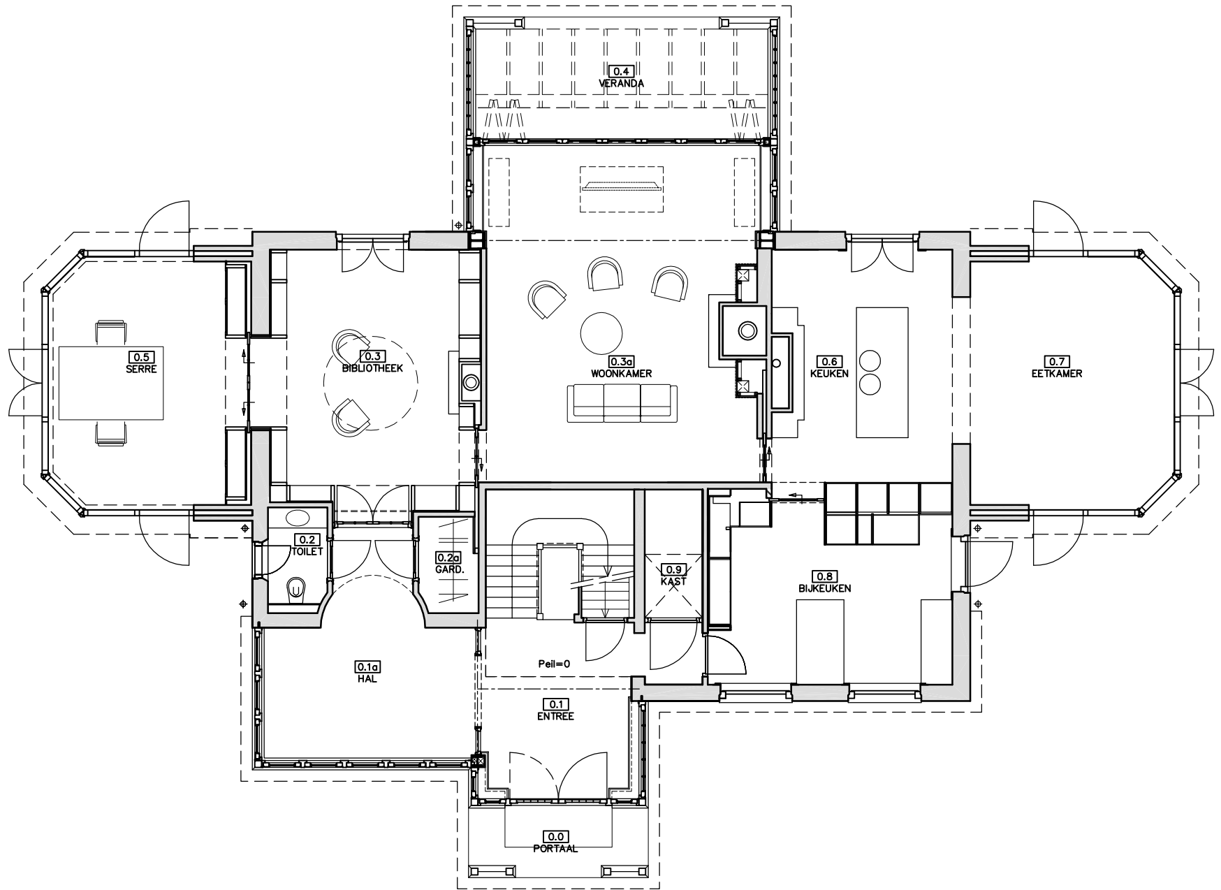
BEGANE GROND
