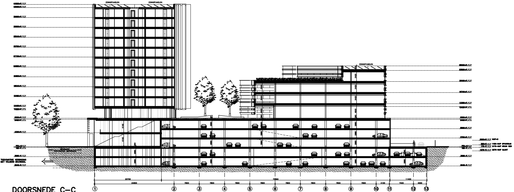
DOORSNEDE C-C
