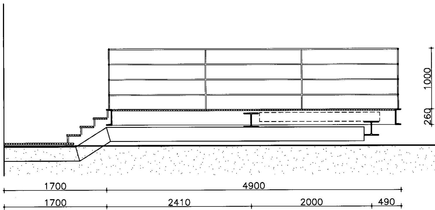
DOORSNEDE TERRAS
