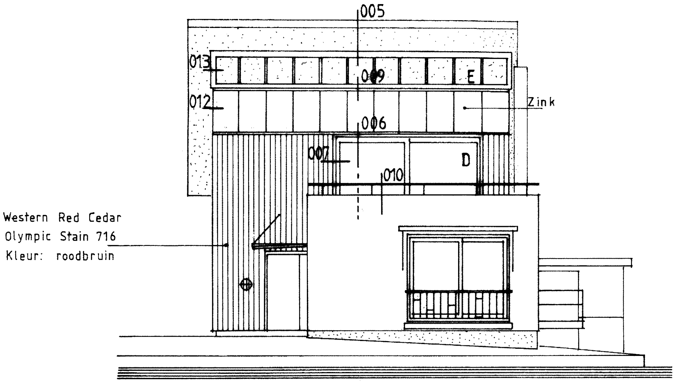
ZUIDGEVEL
