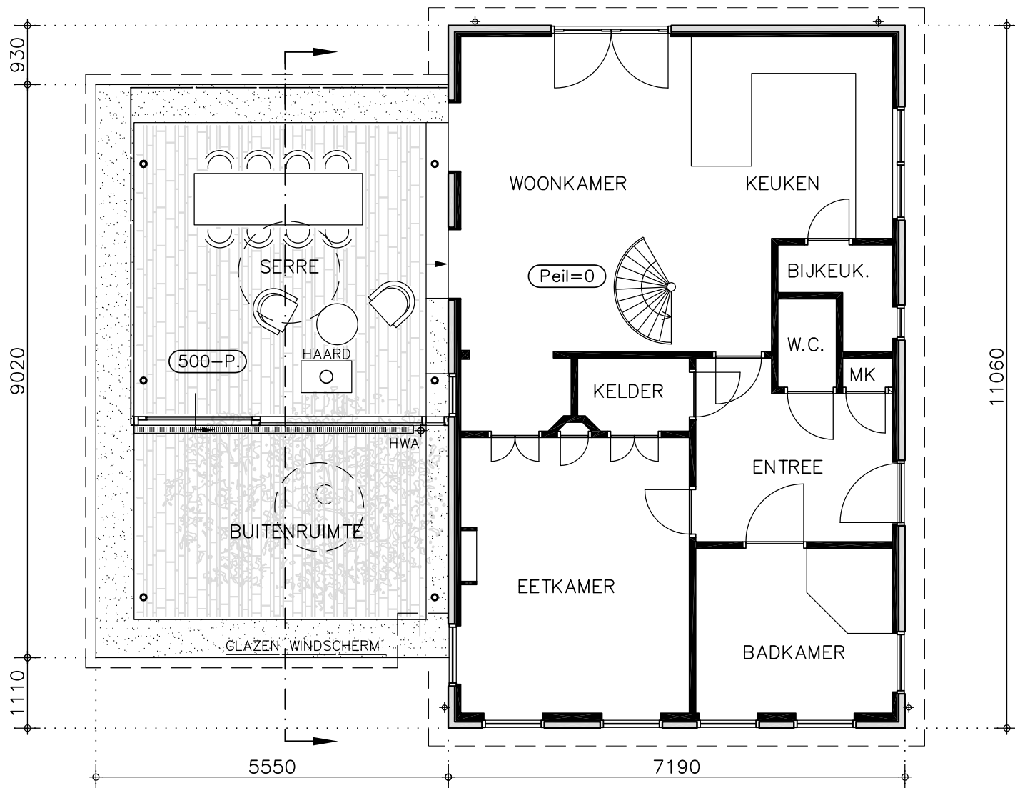
PLATTEGROND
