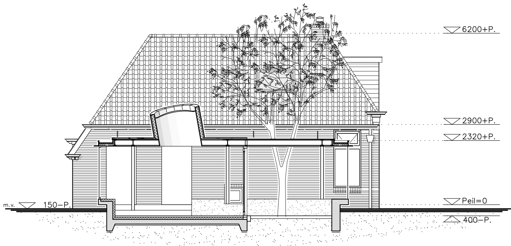
DOORSNEDE
